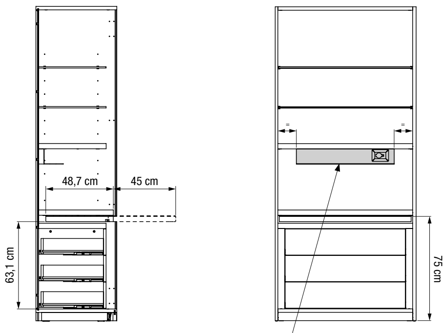
Ripiano accessorizzato da fissare al centro del ripiano. Accessorised shelf to be fastened in the middle of the shelf.
