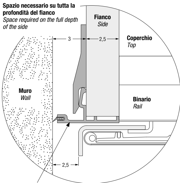
Profilo di tamponamento laccato Lacquered filler profile
